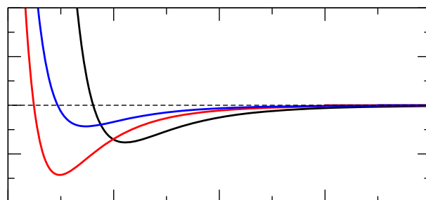
Figur 3. Nikkel-Fosfor modellen. Angivelse af den kraft 3 forskellige par af atomer, Ni-Ni, P-P og Ni-P, kan påvirkes af i modellen. Den største tiltrækningskraft ses her mellem Ni-P, altså mellem Nikkel og Fosfor (rød linje).
